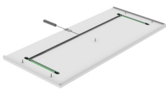
Piastra di sicurezza DIAGO 504 La funzione della piastra di sicurezza è arrestare il movimento del pensile in caso di contatto con qualsiasi oggetto. Scegliere una piastra compatibile con la larghezza del pensile. Da montare sotto il pensile Colore: Bianco Spessore: 12 mm Profondità: 350 mm
